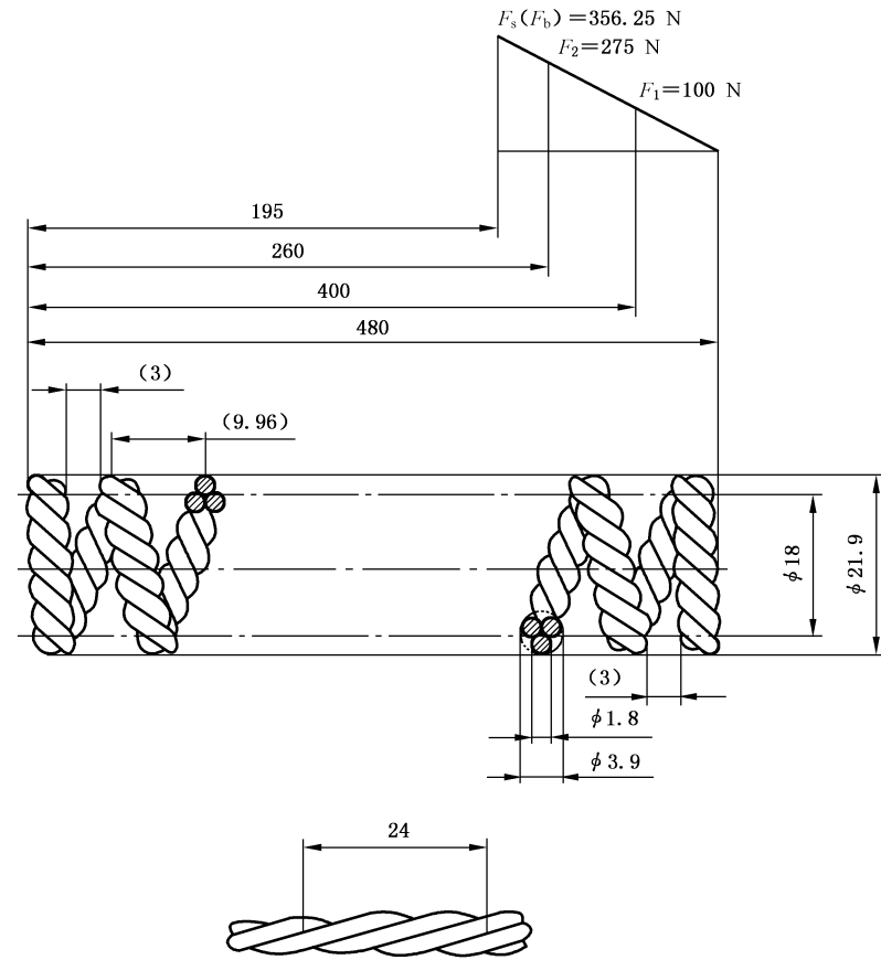
图 A.1 弹簧工作图
